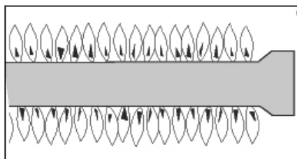
Mauvais réglage : Flammes vives bleues (excès d'air)
